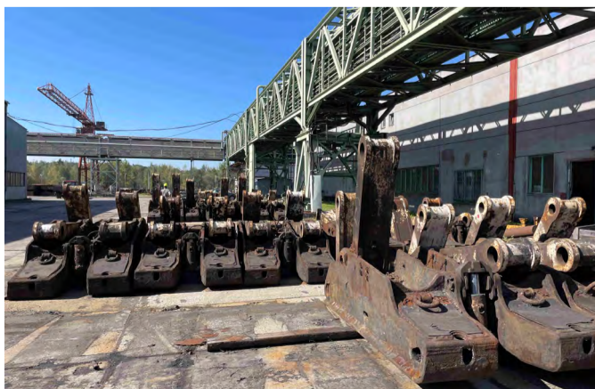
Mechanizované výztuže připravené k nasazení.
