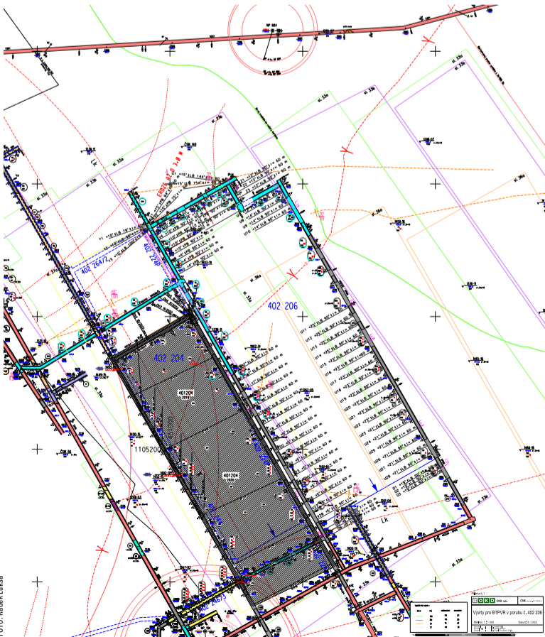
Mapa vývrťů pro BTPVR v porubu 402 206.
